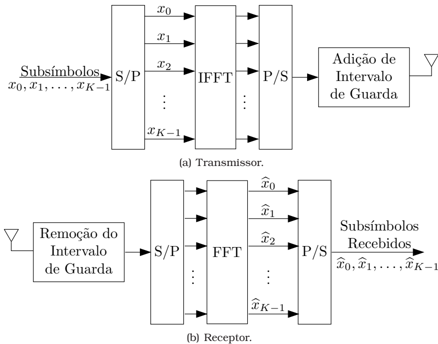
Figura 2.17: Sistema OFDM
