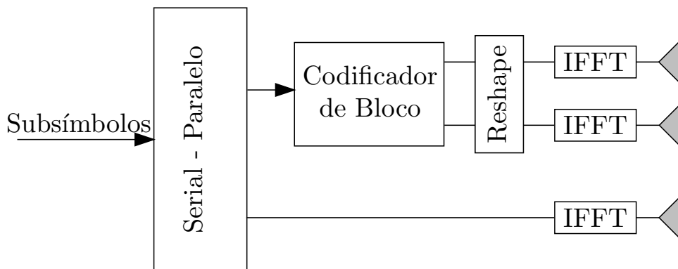
Figura 2.18: Transmissor de um sistema MIMO-OFDM utilizando a estrutura MIMO híbrida apresentada na Figura 2.14.
